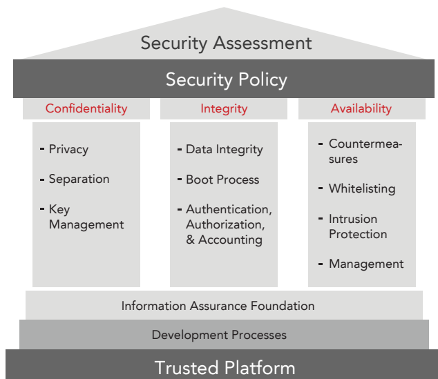
図1: 情報セキュリティの3原則、CIAに基づく Wind River Helix Security Framework
